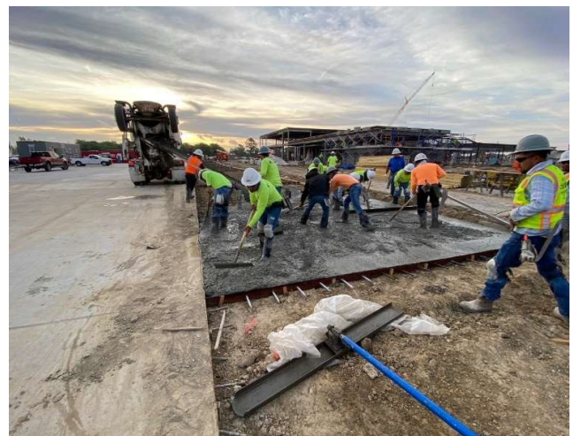
Concrete pour at bus drop-off lane
